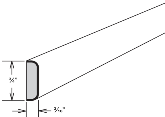
Batten
